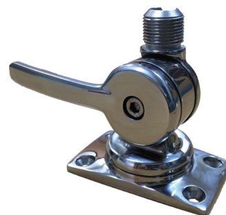
4 VEJS EN-HÅNDS BETJENT rustfri stål dæksbeslag. Ekstra kraftig! Strømlignet udførelse. Patenteret 5 graders justering. 1" 14mm gevind.
