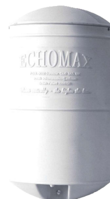
ECHOMAX 230 MIDI Passiv reflektor på 20m 2 . Ideal til RIB's.
